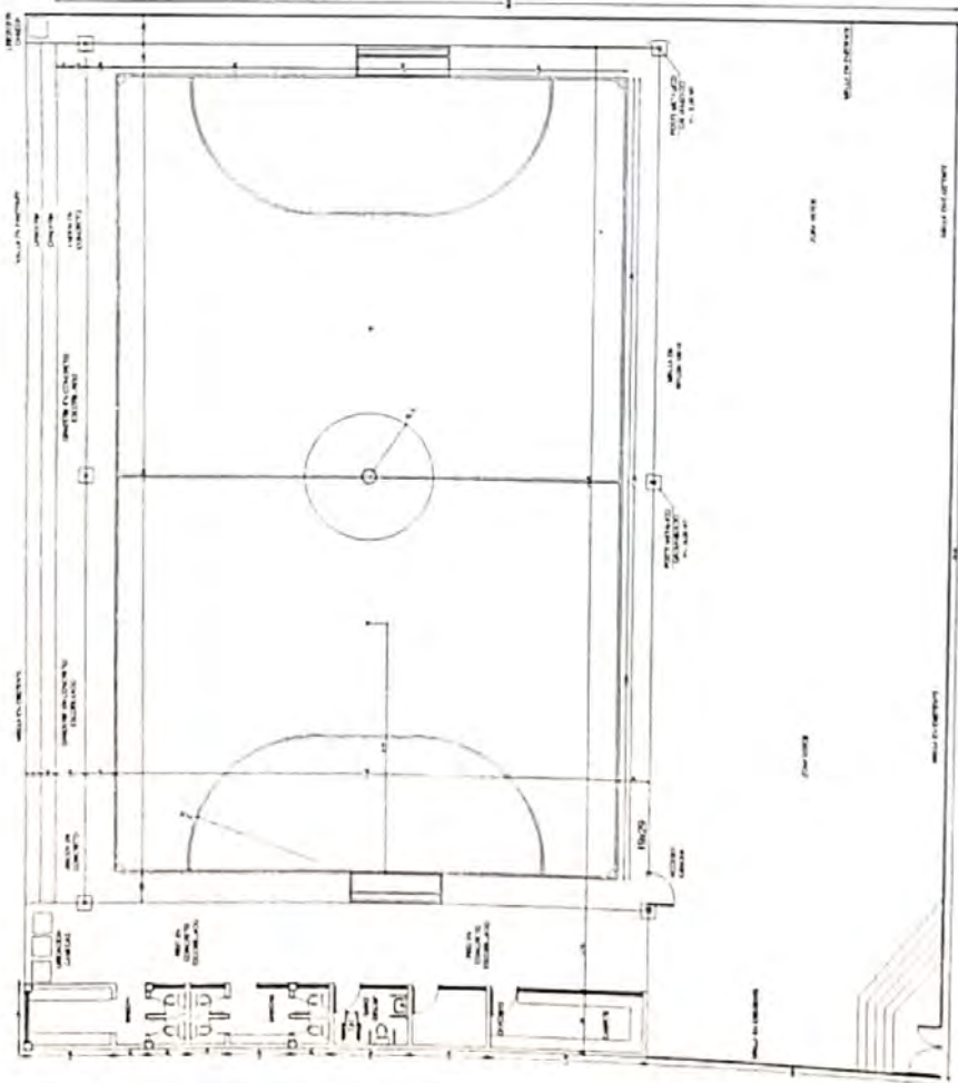
PLANTA CANCHA ESCALA 1:100
